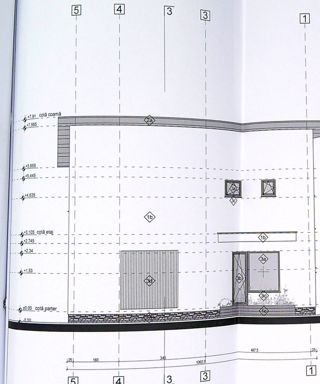
FAȚADĂ EST sc. 1:100
