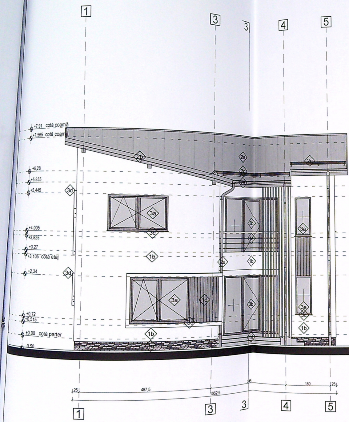
FAȚADĂ VEST sc. 1:100
