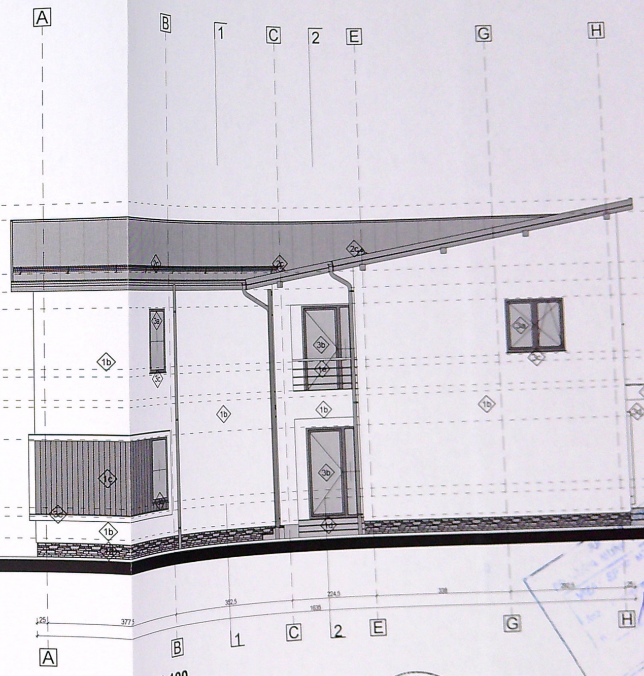
FAȚADĂ SUD sc. 1:100
